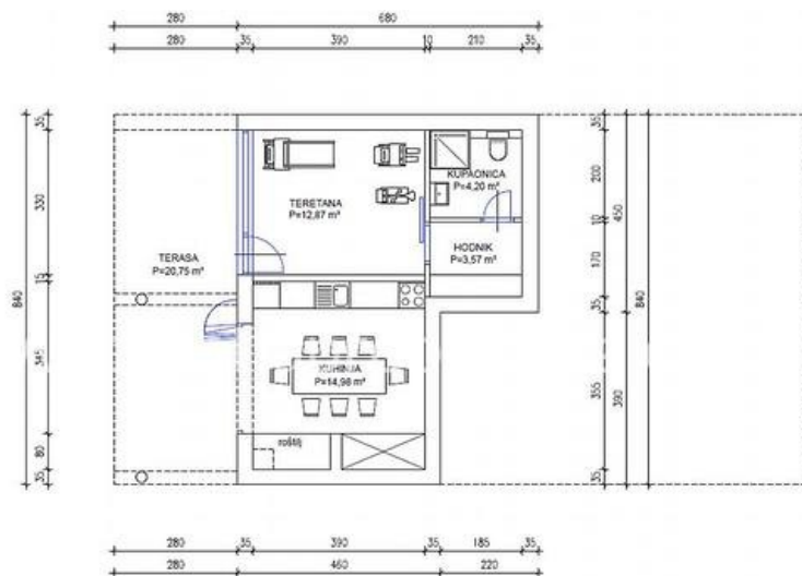
TLOCRT SUTERENA MJ 1:100
