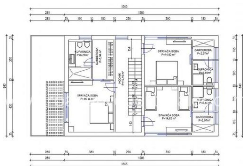
TLOCRT KATA MJ 1:100
